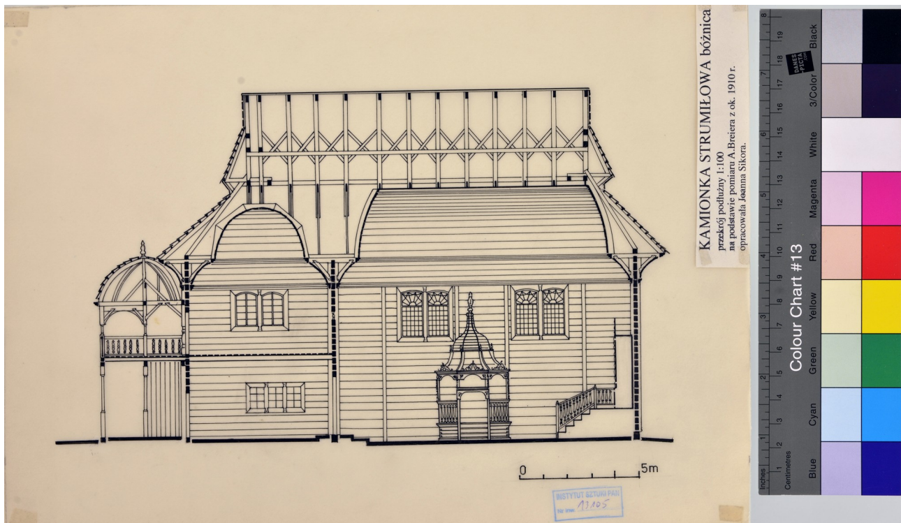
Fig. 4 Longitudinal Section
