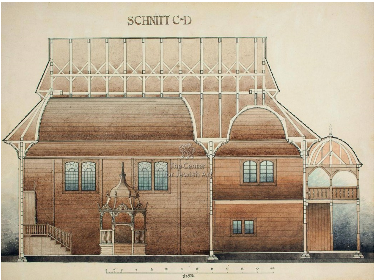
Fig. 13 Longitudinal Section
