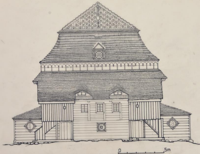
JANÓW SOKÓLSKI bóżnica elewacja zachodnia stan w 1927 1:100
