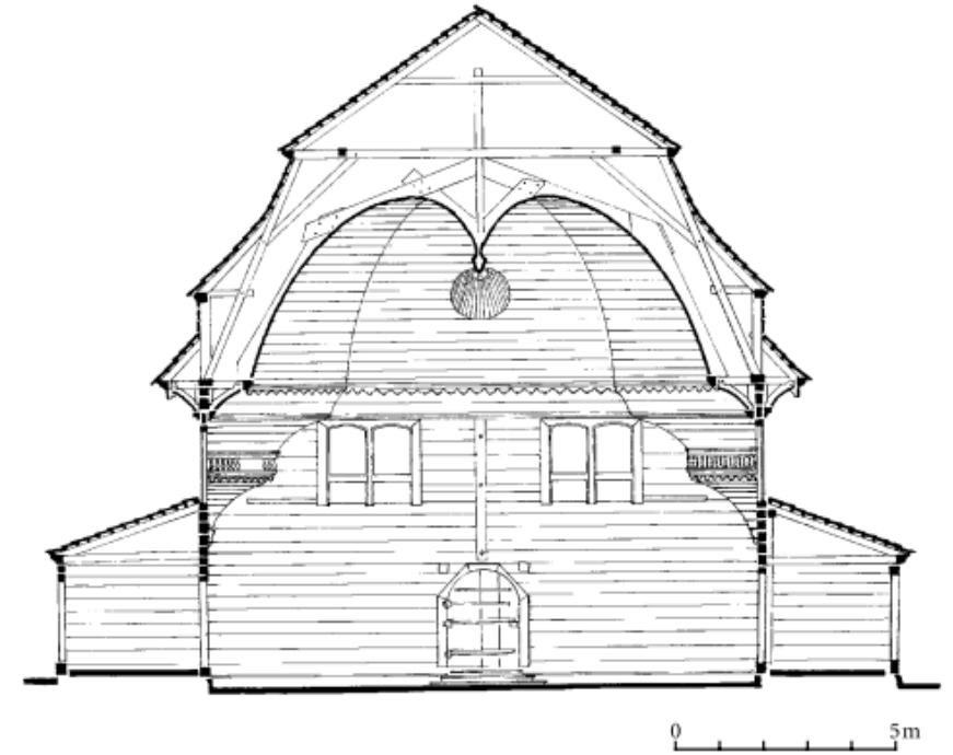
Przekrój poprzeczny z widokiem na ścianę zachodnią
