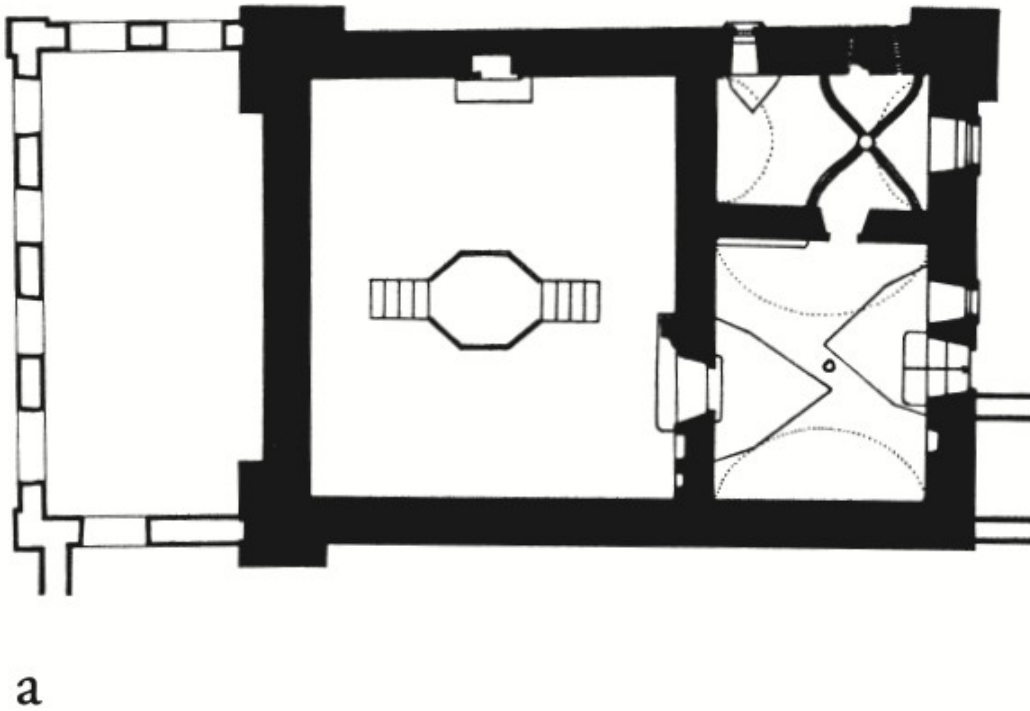
Abb. 15 Grundriss EG
