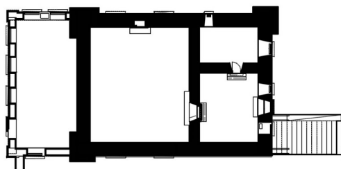
Abb. 29 Grundriss Erdgeschoss
