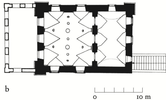
Abb. 21 Grundriss OG
