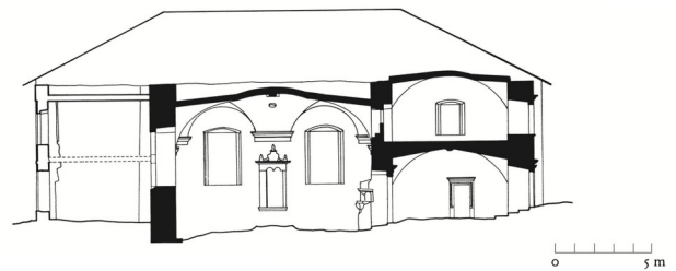
Abb. 19 Schnitt nach Osten
