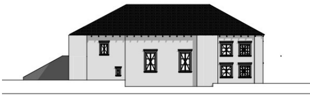
Abb. 23 Ansicht Osten
