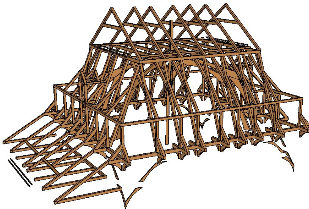
Fig. 58 A.3.1 Główna więźba dachowa
