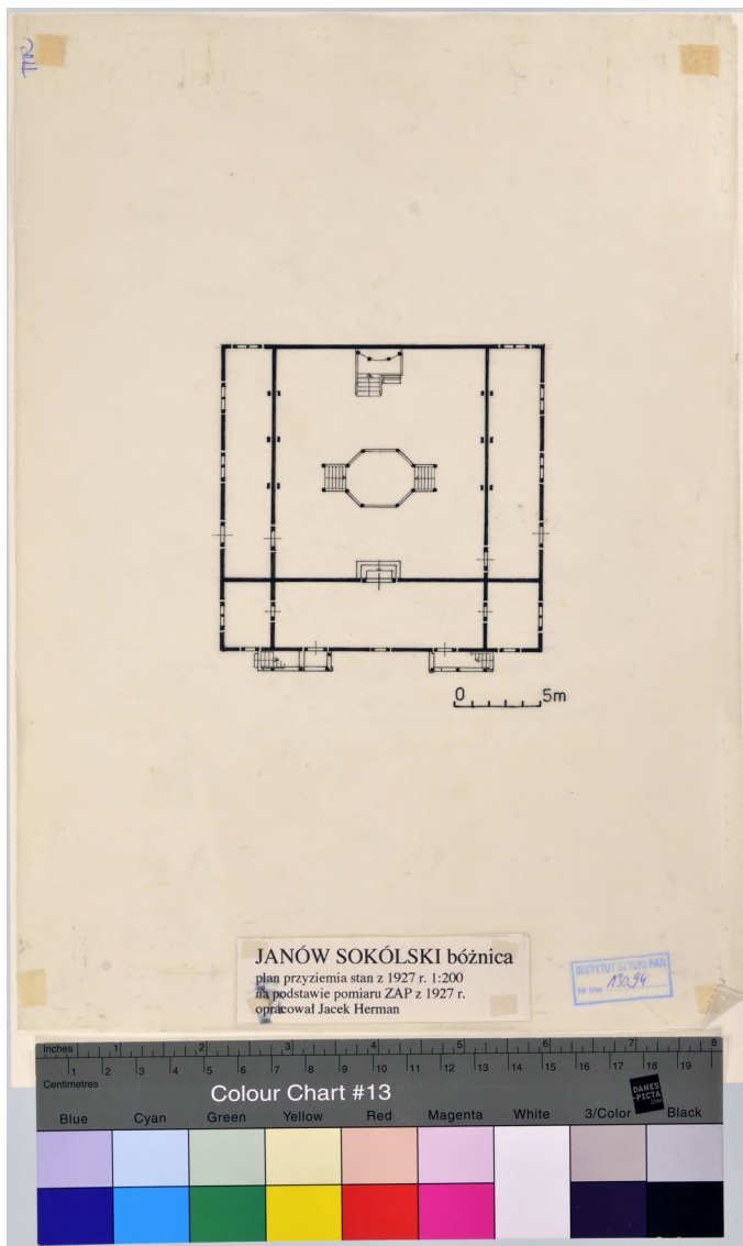
Fig. 5 Rzut z nadbudowanym babińcem
