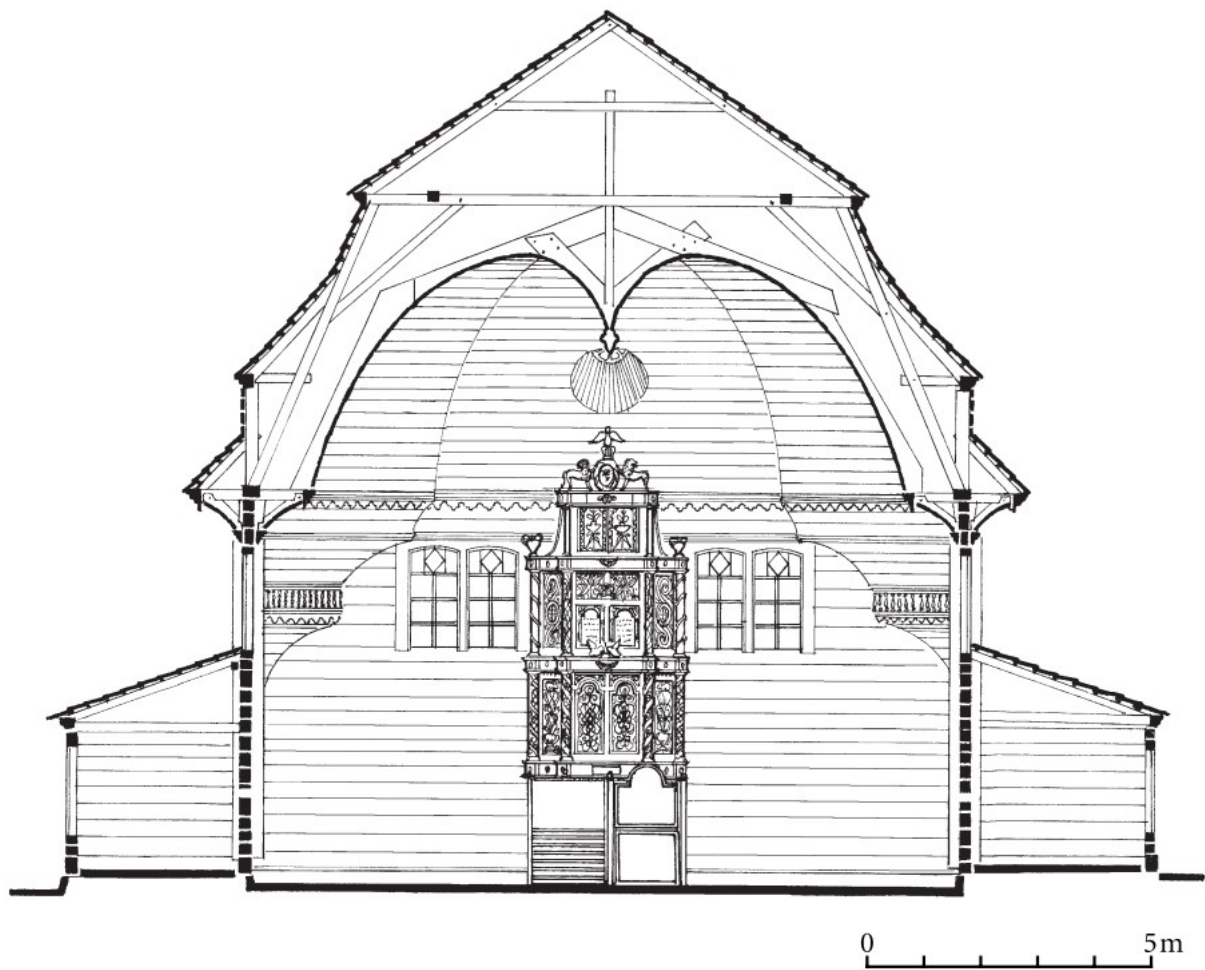
Fig. 25 Przekrój z widokiem na aron ha-kodesz
