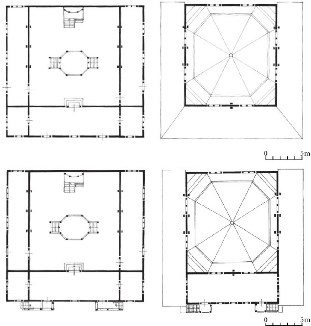
Fig. 18 rzuty kondygnacji i dachów
