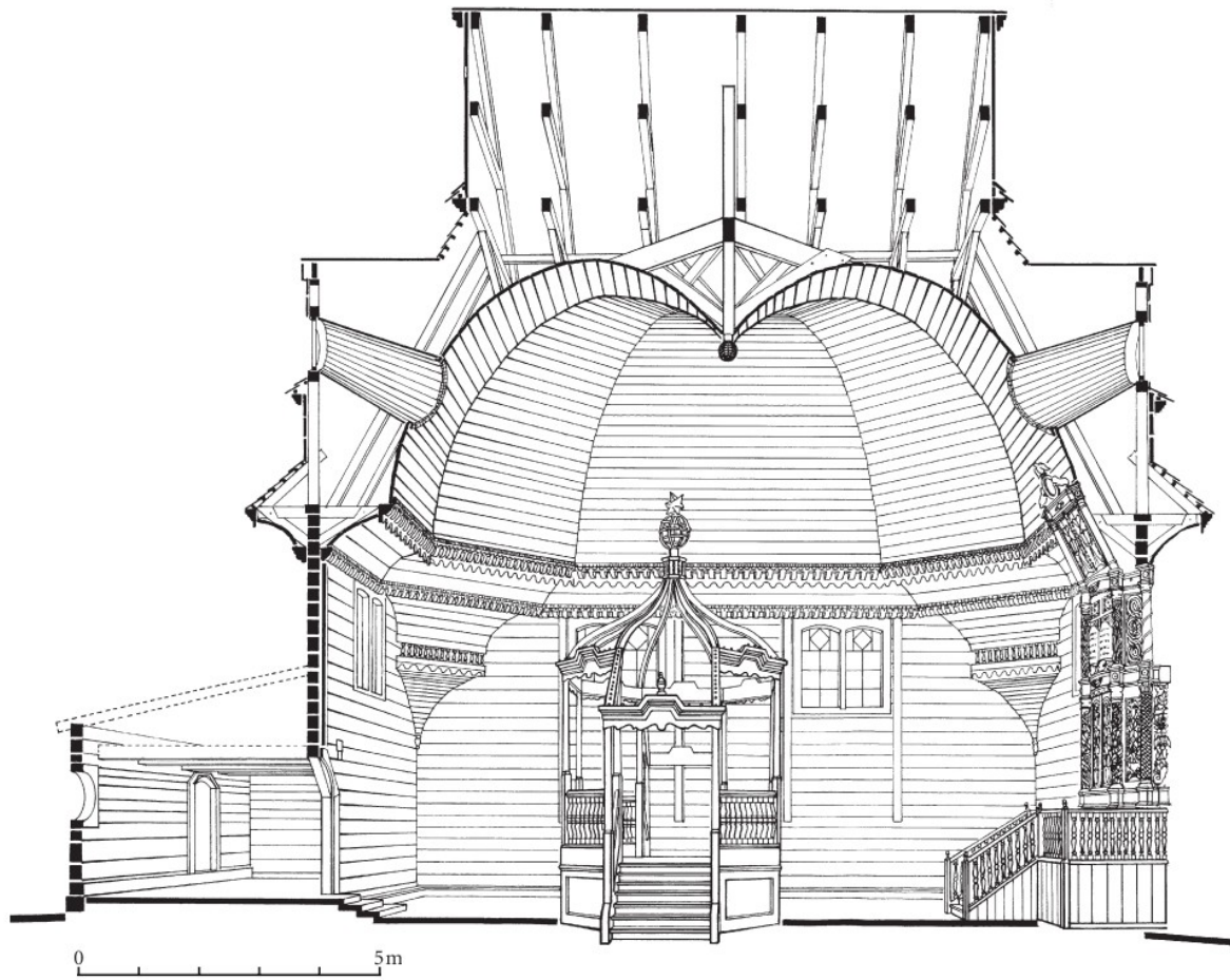
Fig. 14 Przekrój z widokiem na aron ha-kodesz
