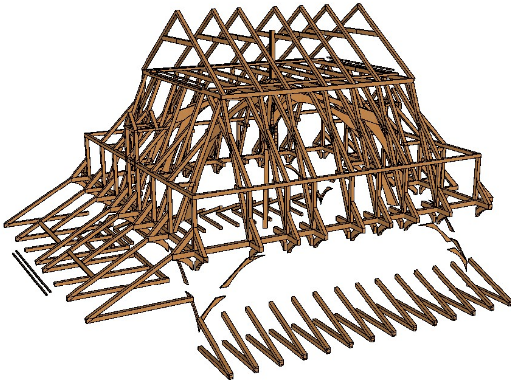
Fig. 57 A.3 Więźba dachowa
