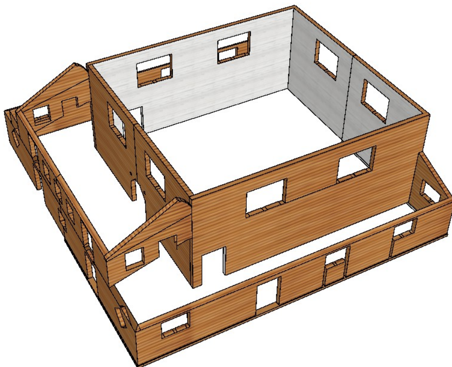
Fig. 60 A.1.1 Ściany nośne
