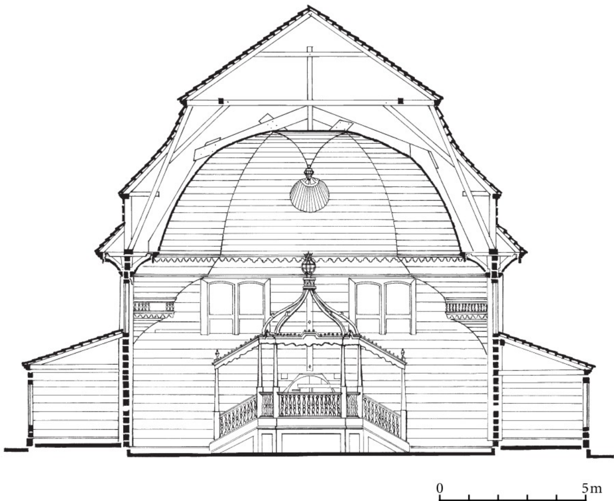
Fig. 8 Widok na elewację zachodnią od wewnątrz wraz z bimą
