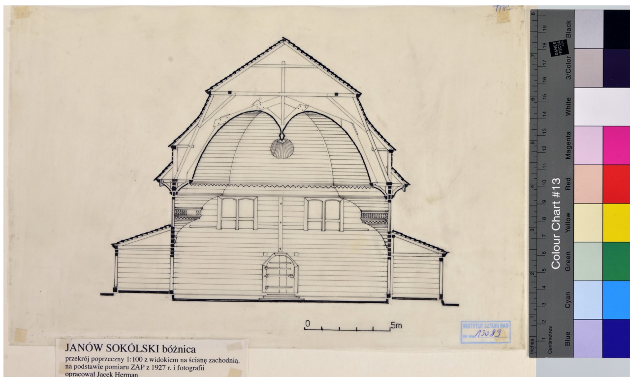
Fig. 7 Widok na elewację zachodnią od wewnątrz
