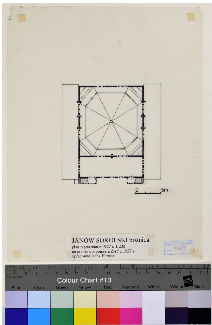
Fig. 4 Rzut dachu po nadbudowie babińca
