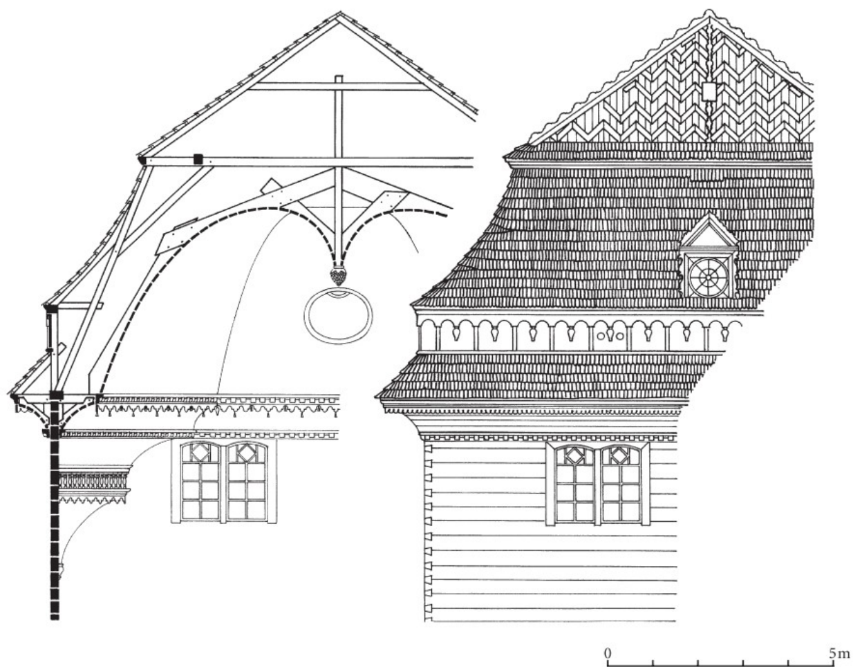
Fig. 13 Elewacja zachodnia i przekrój
