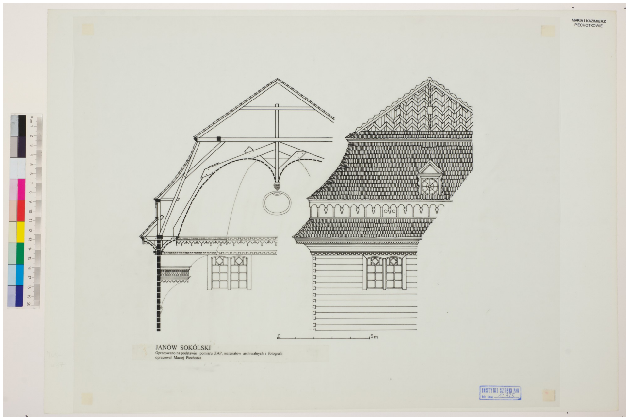
Fig. 32 Elewacja wschodnia i przekrój
