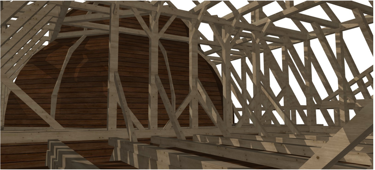
Fig. 137 Dome construction
